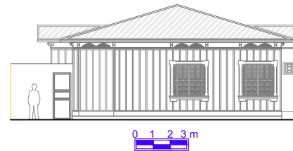
Elevação 03
