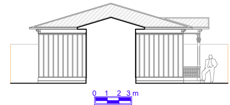
Elevação 04
