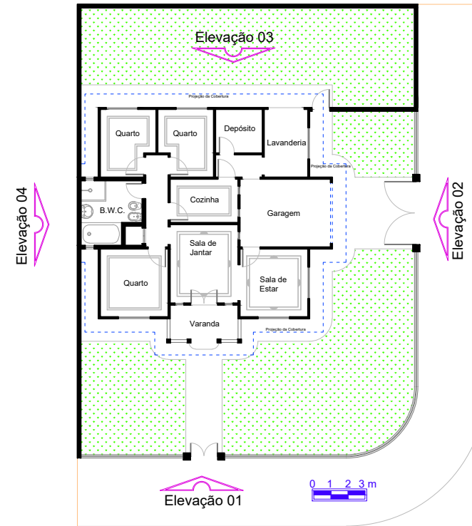
Planta
