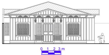
Elevação 01
