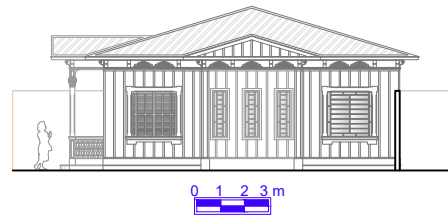
Elevação 02
